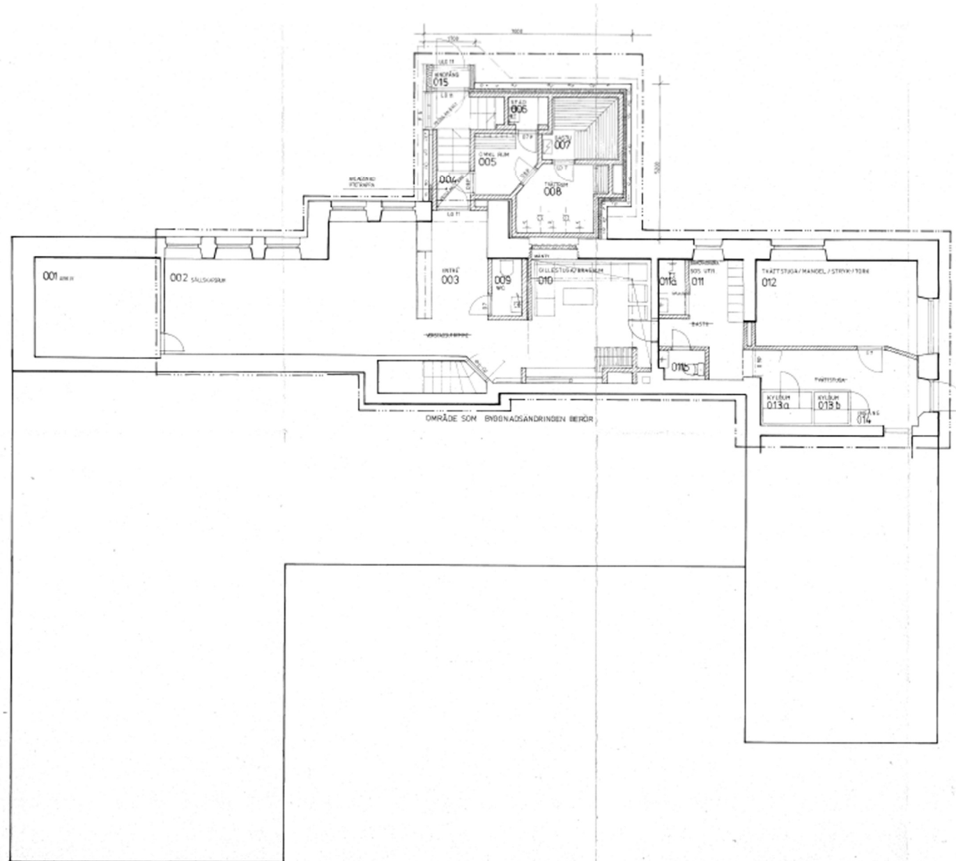
Kuva 7. Päärakennuksen kellarikerros.
