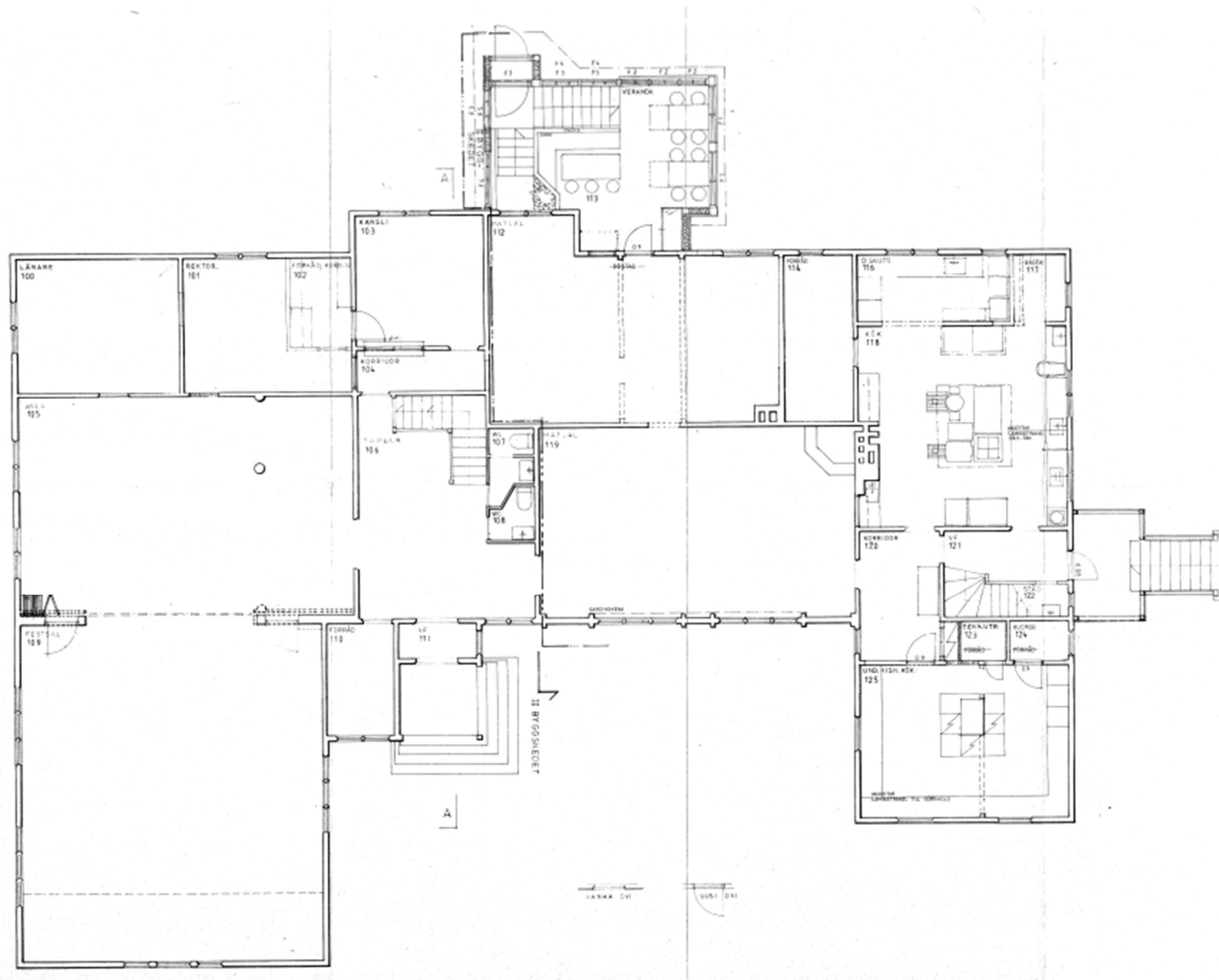
Kuva 8. Päärakennuksen 1. kerros.
